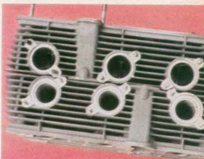
Einlaßtrakte aufgebohrt
