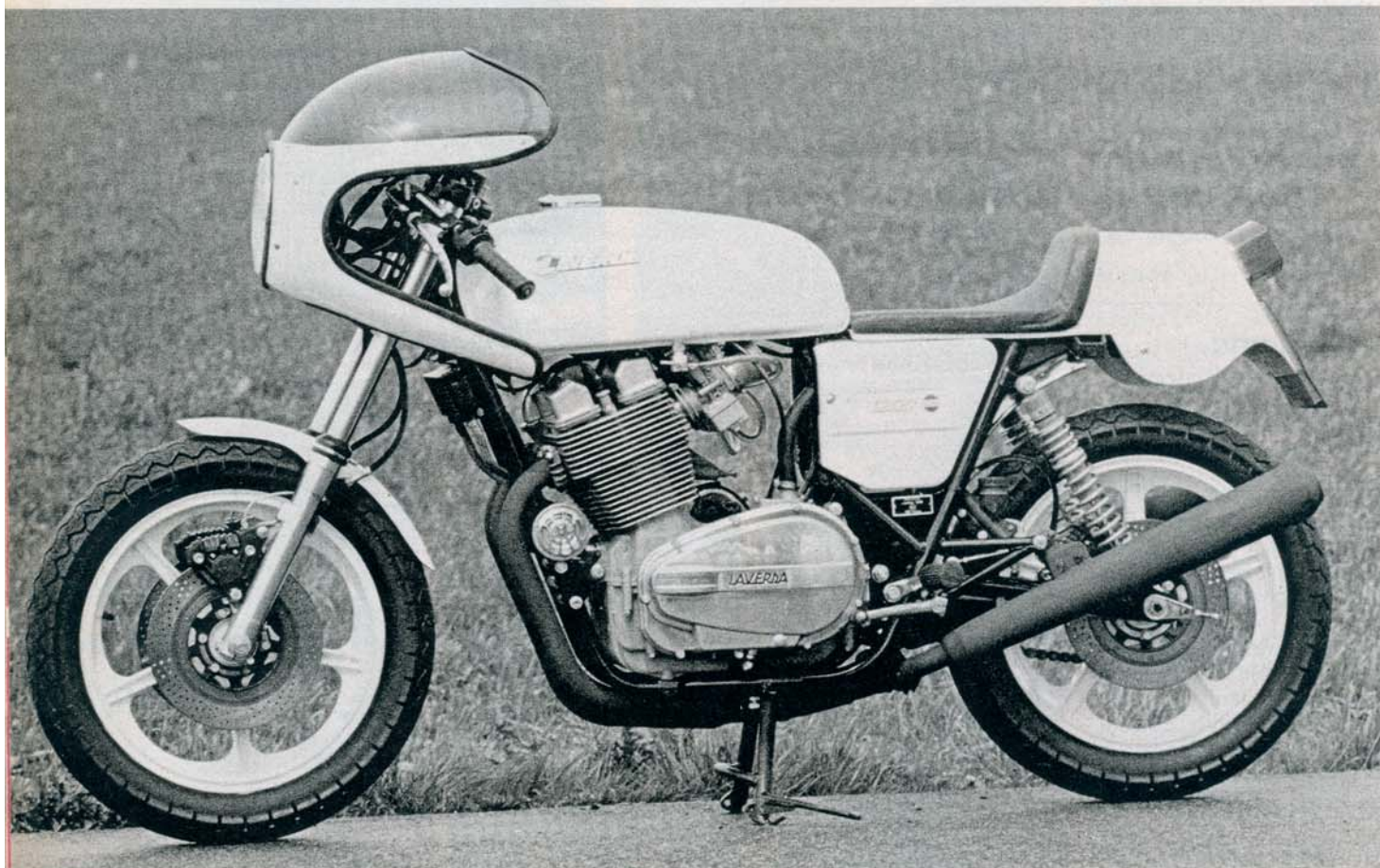
Das Fahrwerk bleibt fast serienmäßig: Hinten dämpfen Bilstein-Gasdruck-Elemente, die Bremsscheiben sind gelocht
